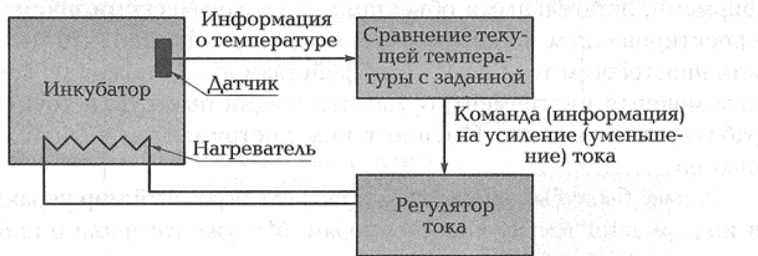
Рис. 2.3. Схема термостата
