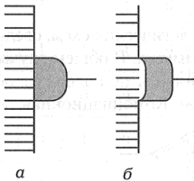
Рис. 3.15. Многовходовые вентили: а — вентиль И; б — вентиль ИЛИ
